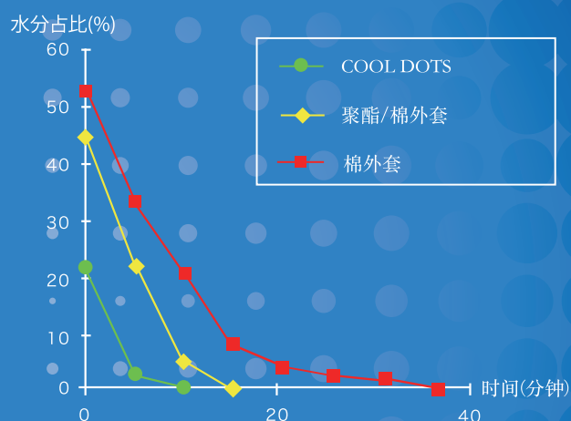
（图1：测定洗涤、脱水后的干燥速度）
